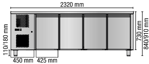
TAVOLO MID GASTRONOMIA / COUNTER MID GASTRONOMY TF04MIDGNSX 4 porte / 4 doors CG - SX Gruppo incorporato a sinistra / Built-in unit on the left side TN Temperatura normale / Normal temperature
