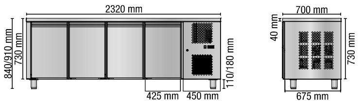
TAVOLO MID GASTRONOMIA / COUNTER MID GASTRONOMY TF04MIDGN 4 porte / 4 doors CG - DX Gruppo incorporato a destra / Built-in unit on the right side TN Temperatura normale / Normal temperature
